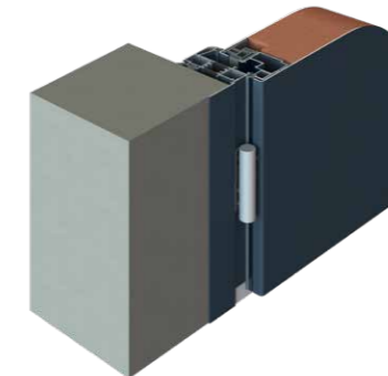
POSE EN BORDS TABLEAU Dormant étroit sans aile + plat de finition
