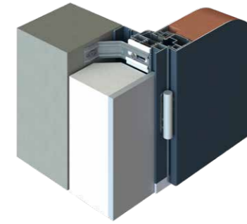
POSE EN APPLIQUE Dormant avec aile de 9 mm + tapée de doublage
