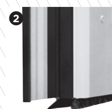
Joints bas EPDM et brosse sur ouvrant
