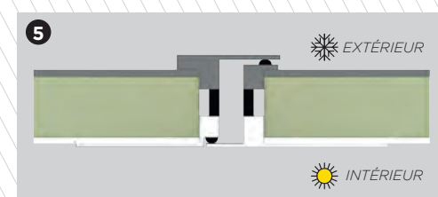
Profils à rupture de pont thermique
