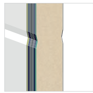
Remplissage panneaux acier et mousse isolante 40 mm
