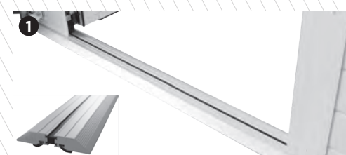
Seuil plat en aluminium (2) (normes PMR) à rupture de pont thermique + 2 joints EPDM
