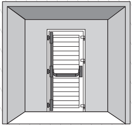
▲ Barre anti-panique (ouverture extérieure uniquement)
