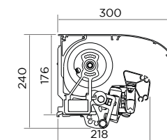
Perle et Perle Lux Pose Face avec auvent
