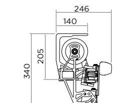
Jade bras croisés Pose Plafond
