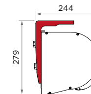
Rubis & Rubilux - Pose plafond -
