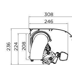
Jade avec auvent Pose Face
