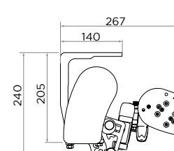
Perle Volant Pose Plafond
