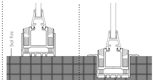
Rail posé au sol standard
